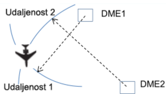
Slika 3.5. Preletištae dobiveno sjecišten dvije DME udaljenosti Izvor: [11]
