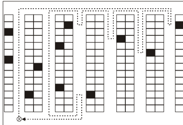
Slika 13. Prikaz optimalnog algoritma za kretanje komisionera [14]
