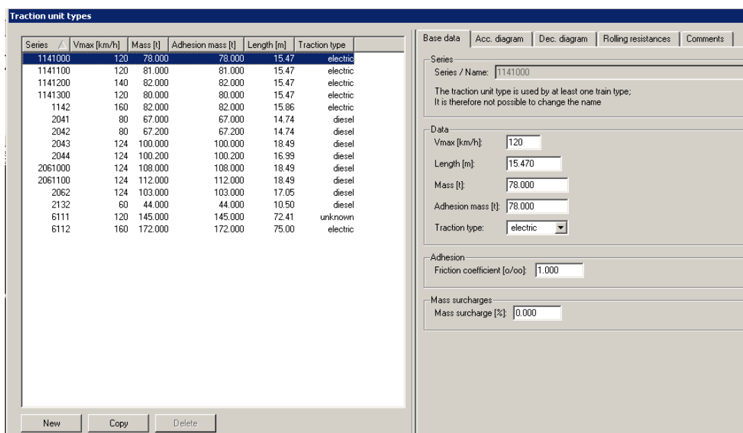
Slika 10. Postupak izrade vučnog vozila
