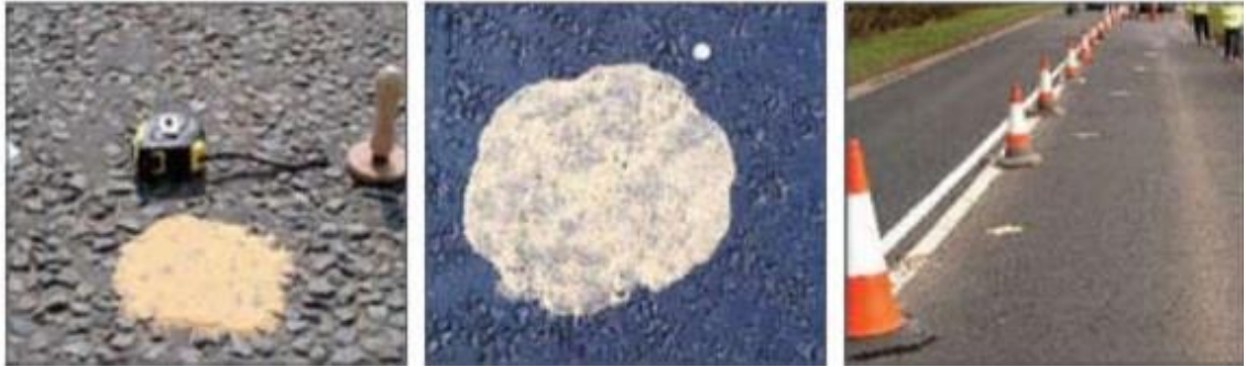
Slika 20. Određivanje dubine teksture pjeskarenjem
