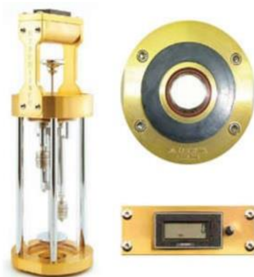
Slika 21. Outflow Meter
