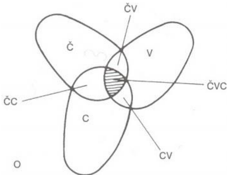
Slika 1. Vennov dijagram
