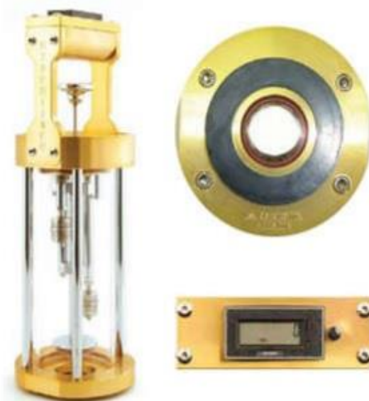
Slika 21. Outflow Meter
