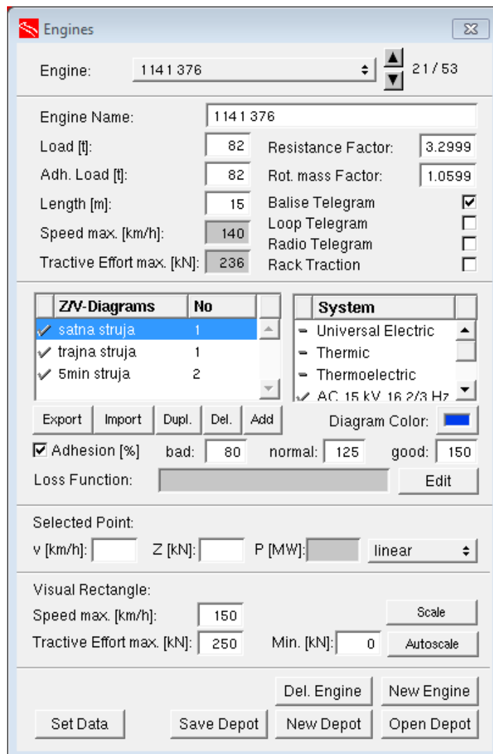
Slika 2.10. Prozor s unesenim podacima za lokomotivu serije HŽ 1141 376
