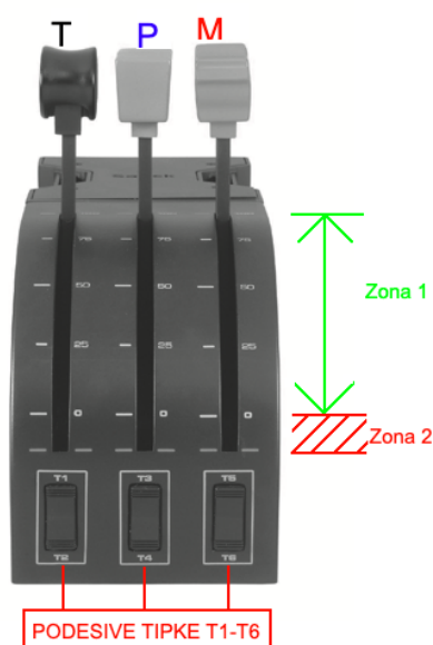
Slika 6 Prikaz ručica snage-propelera-smjese [5]
