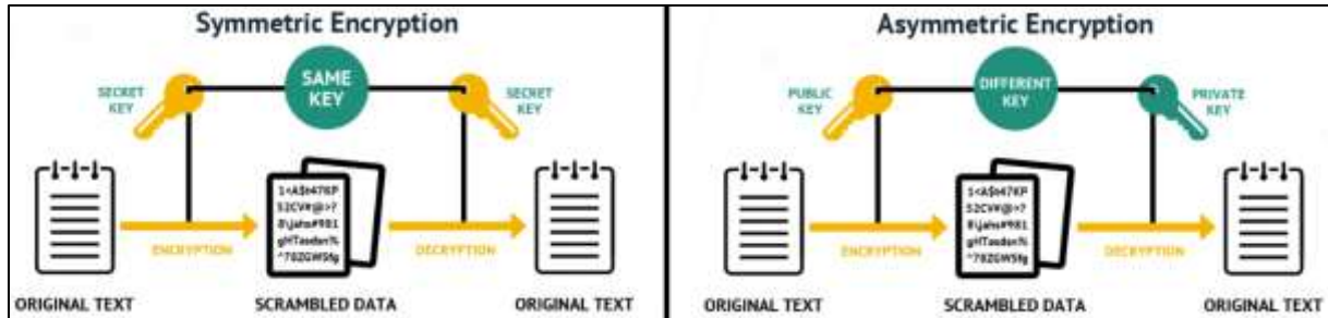
Slika 4: Usporedba procesa enkripcije sa simetričnim i asimetričnim ključem
