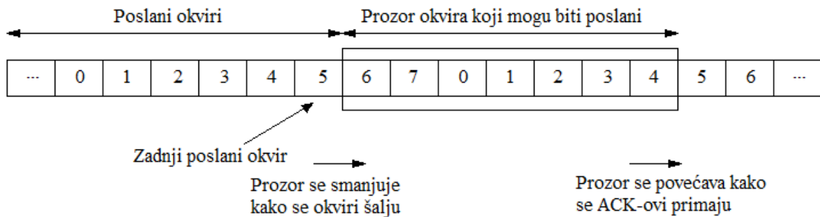
Slika 2. Okviri koji se šalju sa stajališta pošiljatelja, [6]
