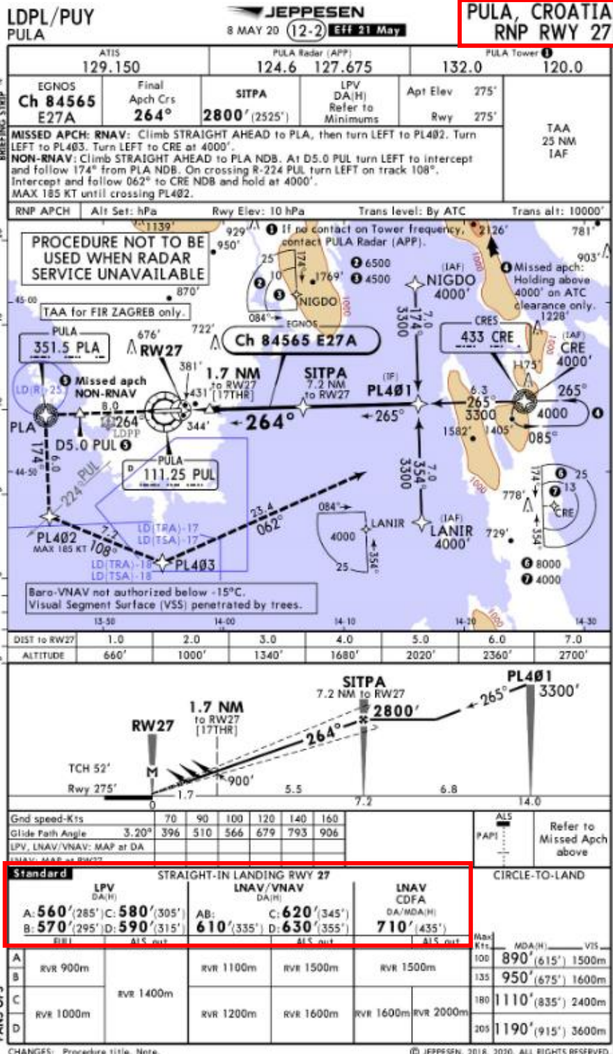
Slika 4.4. RNP postupak prilaznja definiran za USS 27 smještenu u Puli, [7]
