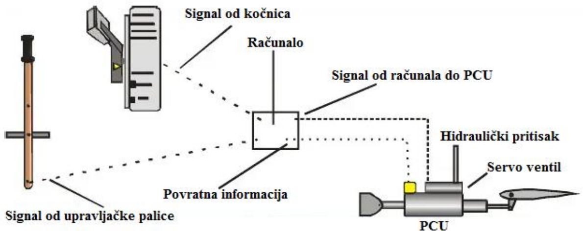
Slika 35.: Osnovni prikaz "Fly by wire" sustava upravljanja zrakoplovom [1]
