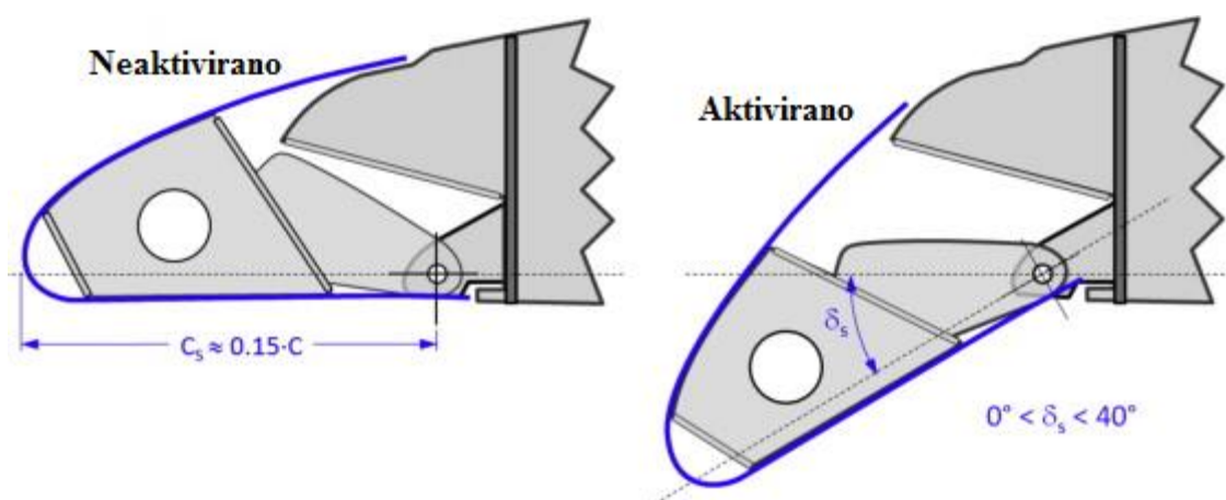
Slika 12.: Zakretni nos pretkrilca
