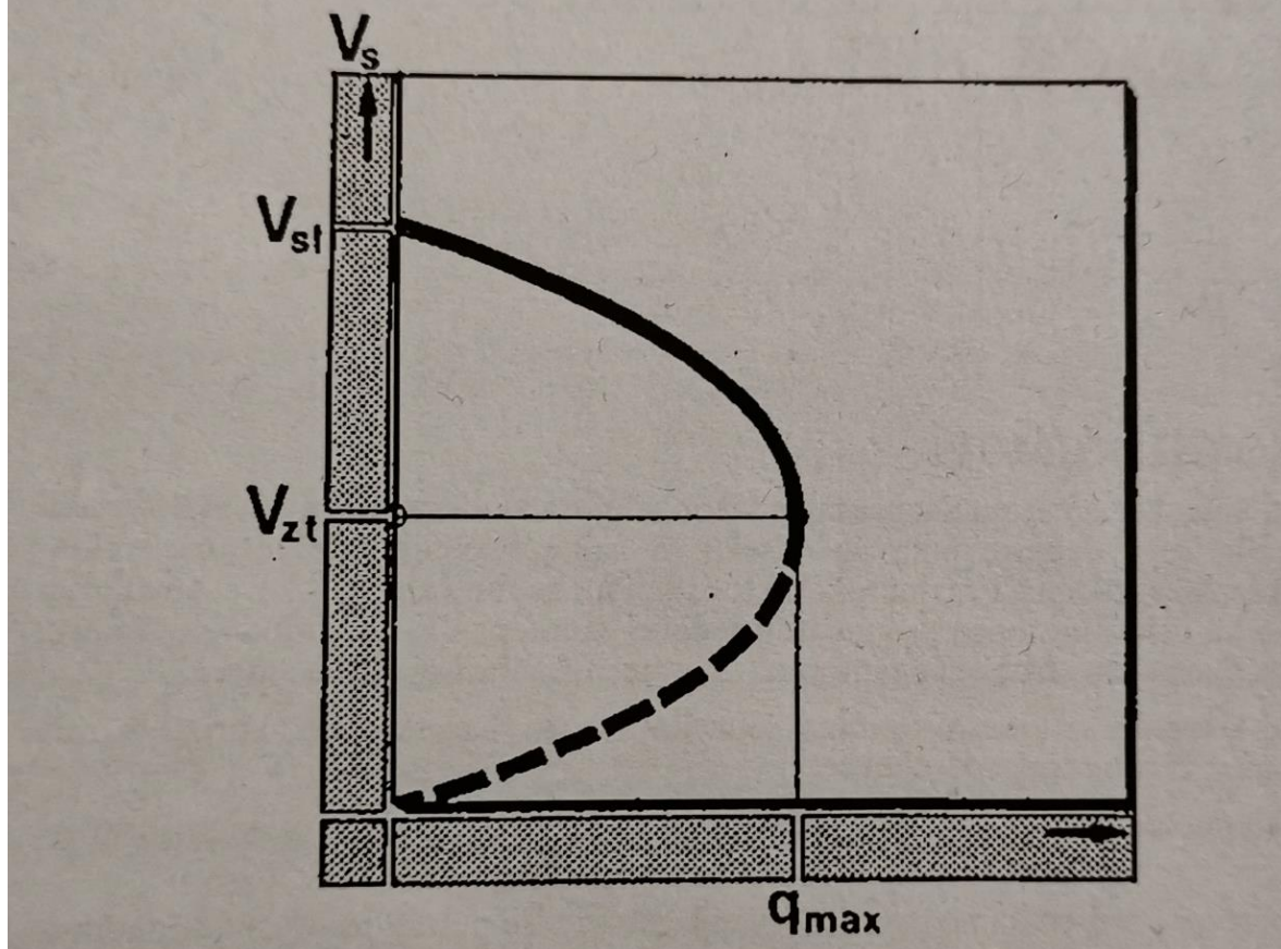
Slika 9. Ovisnost srednje prostorne brzine toka o protoku [7]
