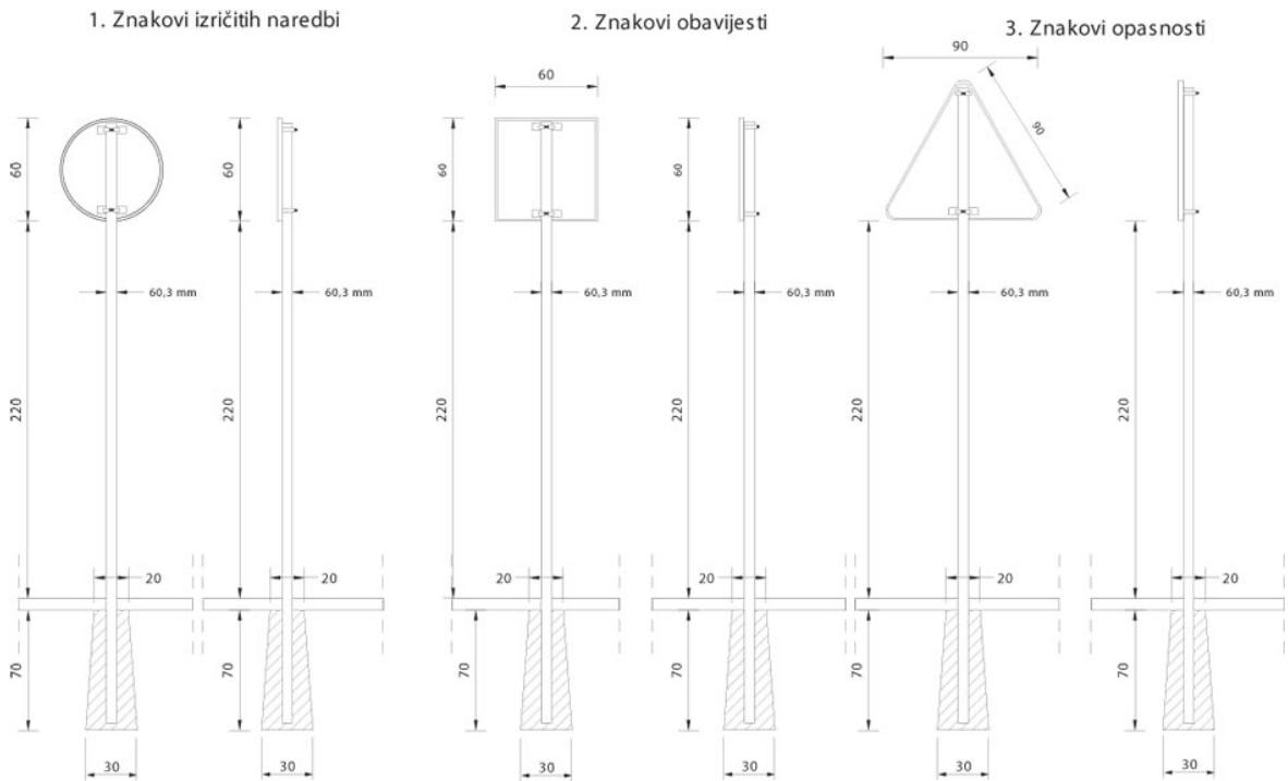
Slika 8. Grafički prikaz pravilnog postavljanja prometnih znakova
