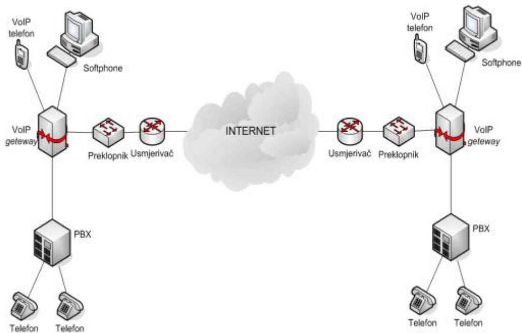
Slika 1. VoIP arhitektura, [4]
