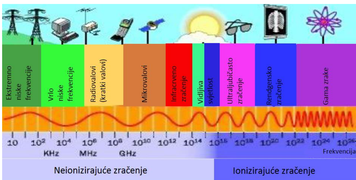
Slika 11. Elektromagnetski spektar [14]
