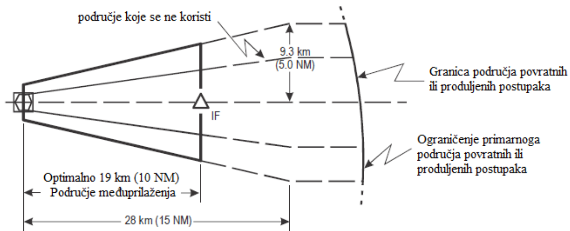
Slika 6. Segment međuprilaženja unutar povratnih i produženih postupaka s preletištem
