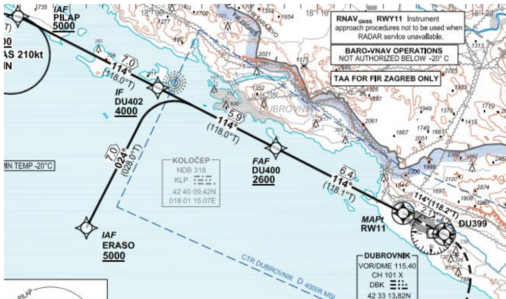
Slika 26. Aerodrom Dubrovnik – isječak iz prilazne RNAV (GNSW) karte za stazu 11
