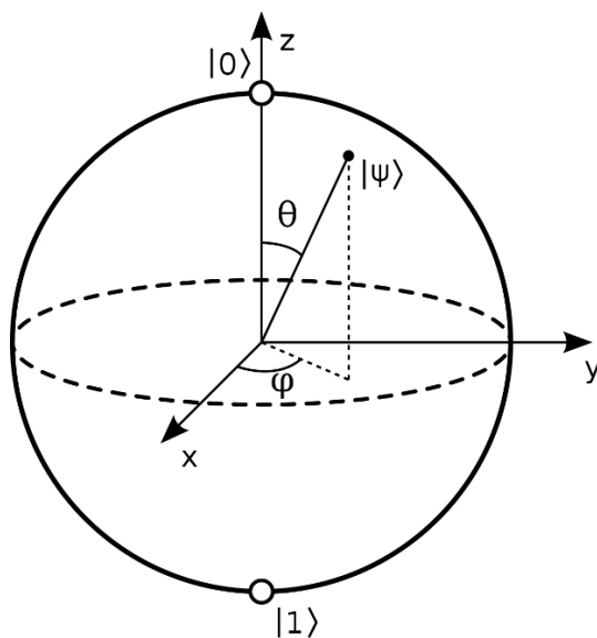
Slika 1. Bloch-ova sfera [2]
