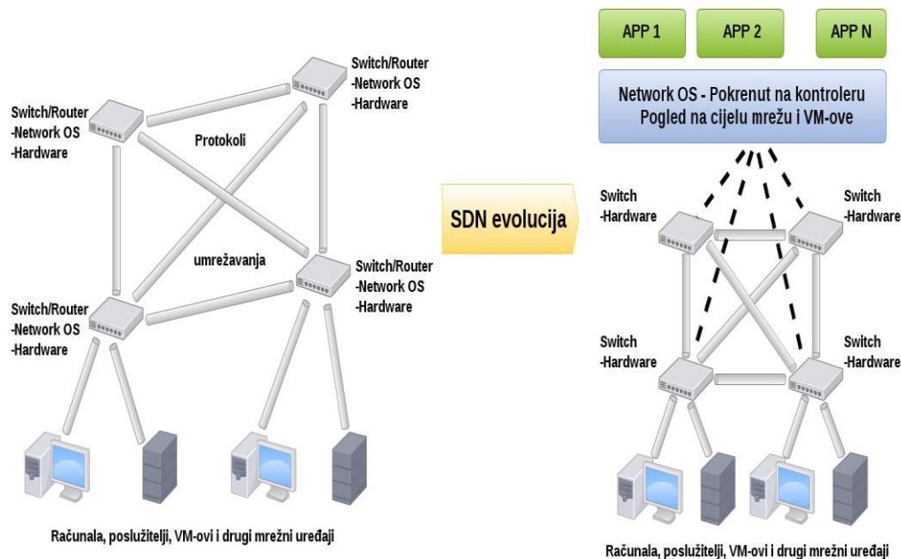
Slika 1. Definicija konvencionalne mreže i definicija SDN-a iste mreže
