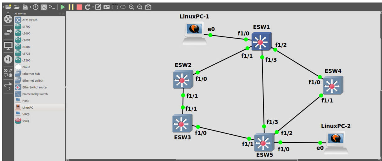
Slika 28. Mrežna topologija konvencionalne mreže u GNS3 simulatoru
