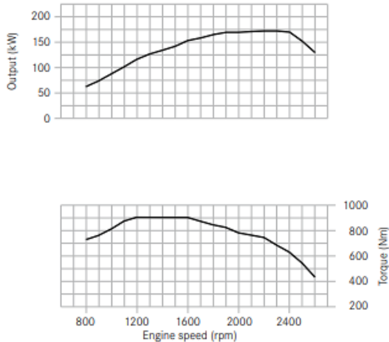
Slika 11: Krivulja snage i okretnog momenta teretnog motornog vozila marke Mercedes-Benz motora snage 170 kW (231 KS)
