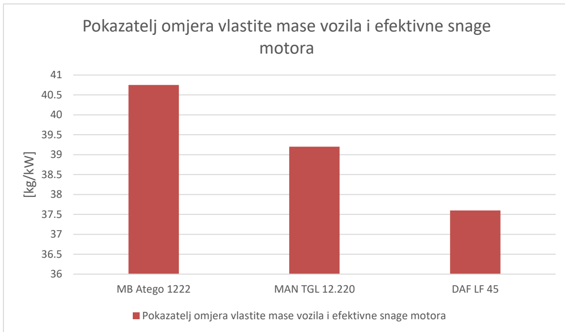
Grafikon 3: Pokazatelj omjera vlastite mase vozila i efektivne snage teretnih motornih vozila marke Mercedes-Benz modela Atego 1222, marke MAN modela TGL 12.220 i marke DAF modela LF 45
