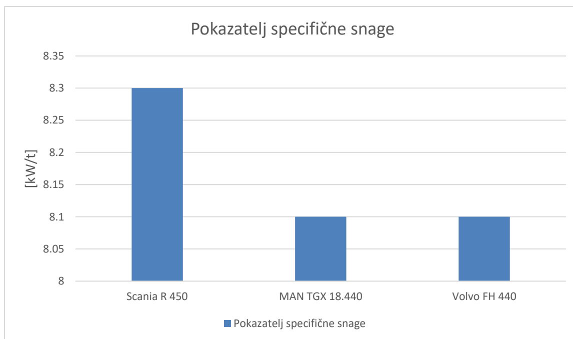
Grafikon 5: Pokazatelj specifične snage teretnih motornih vozila marke Scania modela R 450, marke MAN modela TGX 18.440 i marke Volvo modela FH 440
