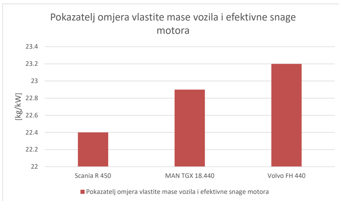
Grafikon 6: Pokazatelj omjera vlastite mase vozila i efektivne snage teretnih motornih vozila marke Scania modela R 450, marke MAN modela TGX 18.440 i marke Volvo modela FH 440
