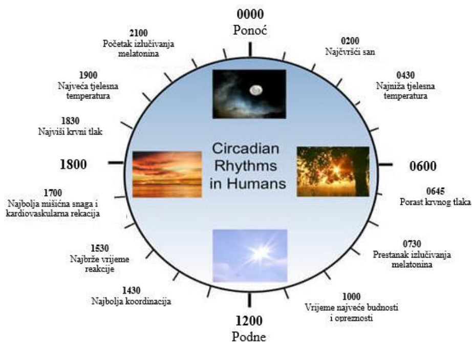
Slika 4. Cirkadijski ritam, [26]
