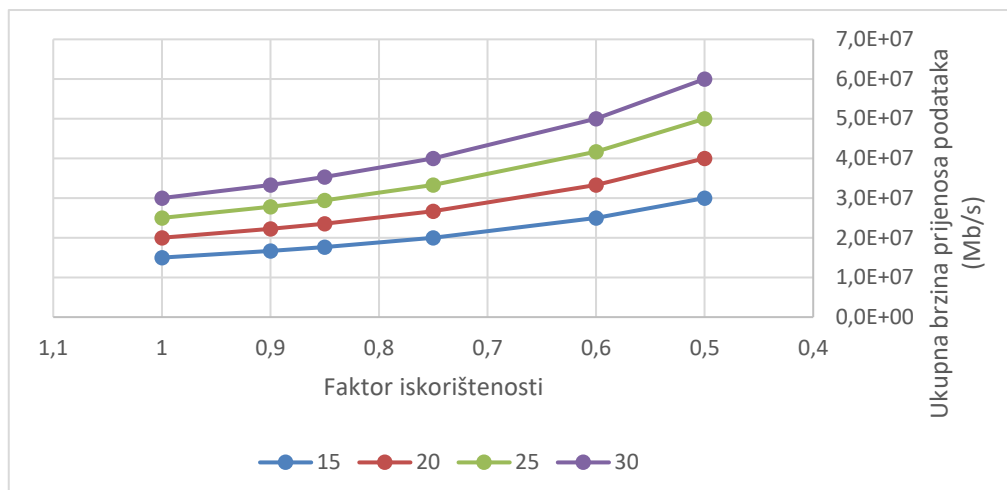
Grafikon 1. Odnos ukupne brzine prijennosa podataka, prosječne brzine i faktora iskorištenosti
