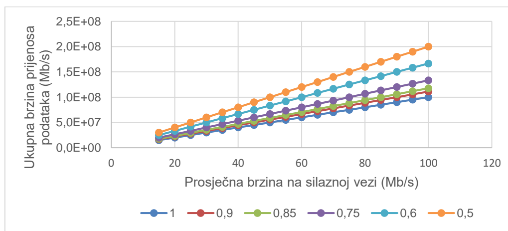
Grafikon 2. Odnos ukupne brzine prijennosa podataka, prosječne brzine na silaznoj vezi i faktora iskorištenja
