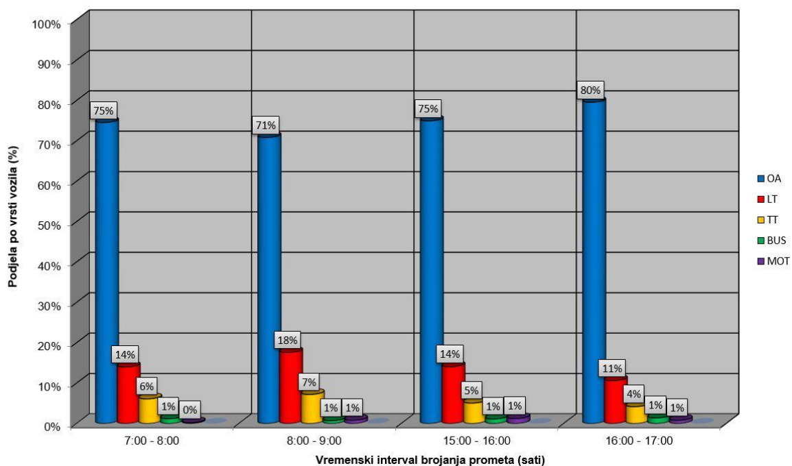
Grafikon 4. Postotak vozila po kategorijama (osobni automobil-OA, lako teretno vozilo-LT, teško teretno-TT, autobus-BUS, motocikl-MOT)
