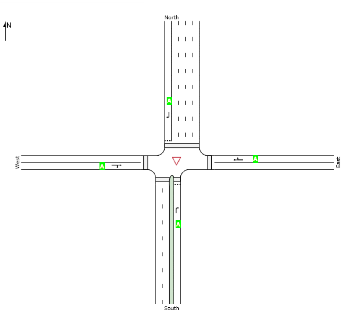
Slika 35. Razina usluge drugog varijantnog rješenja
