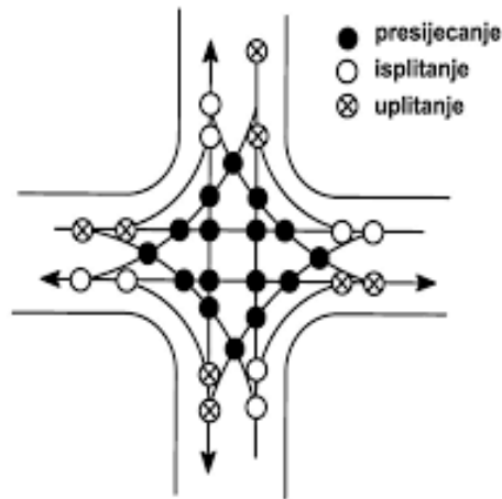
Slika 14. Prikaz konfliktnih točaka [9]
