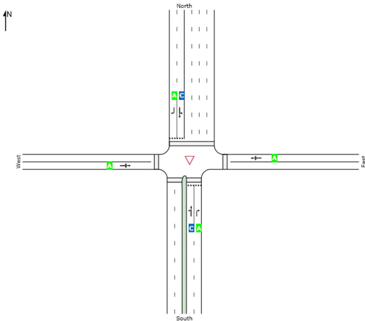
Slika 33. Prikaz razine usluge prve varijante u programskom alatu Sidra Intersection
