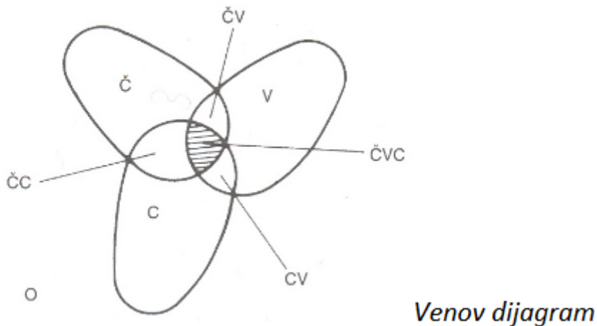
Slika 1. Vennov dijagram [1]
