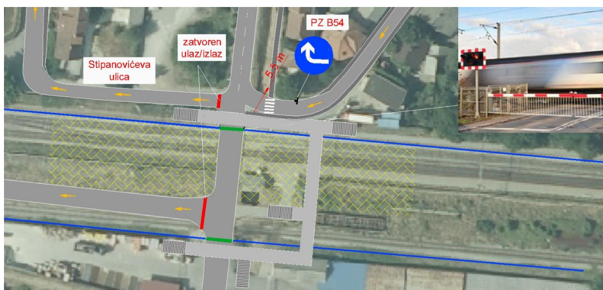
Slika 16. Pozicija predviđene prometne opreme na ŽCP-u Sokolska
