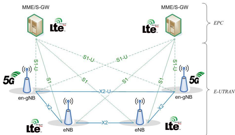
Slika 16. NSA Arhitektura, [10]
