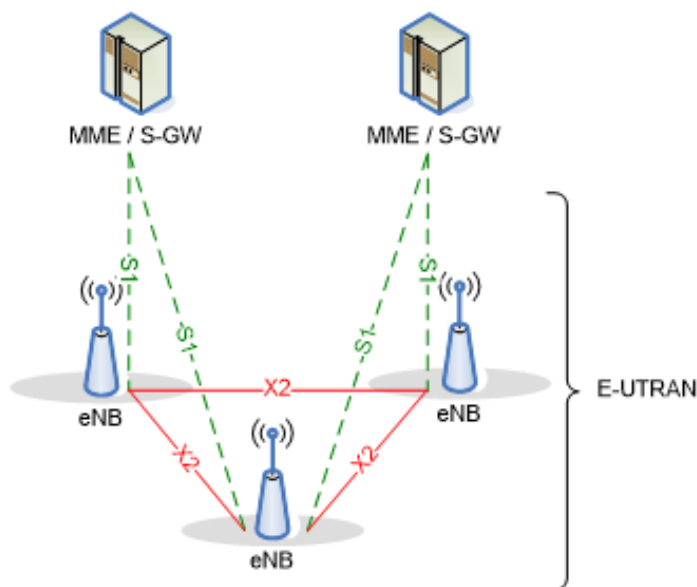
Slika 12. E-UTRAN Arhitektura, [14]
