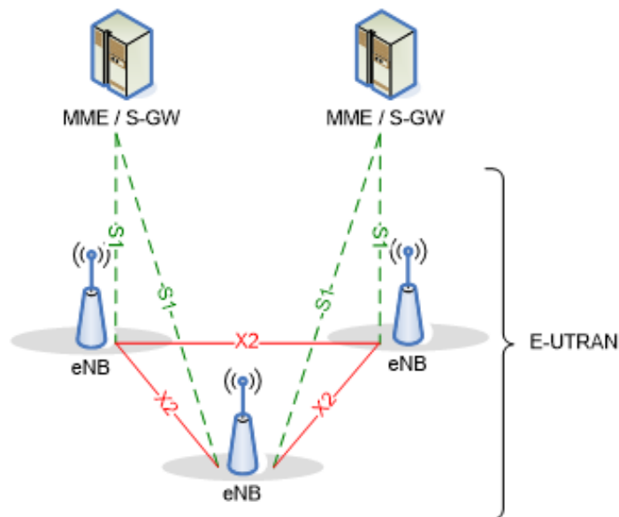
Slika 12. E-UTRAN Arhitektura, [14]
