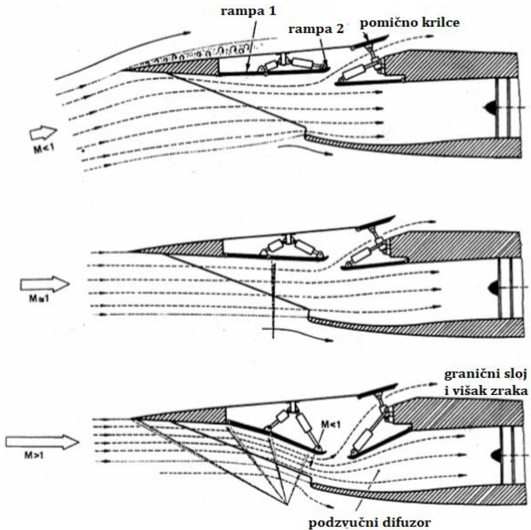
Slika 6 - Ravninski uvodnik [3]
