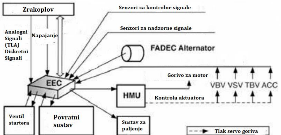
Slika 18 - FADEC sustav [9]
