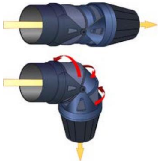
Slika 26 - Mlaznik STOVL motora [10]
