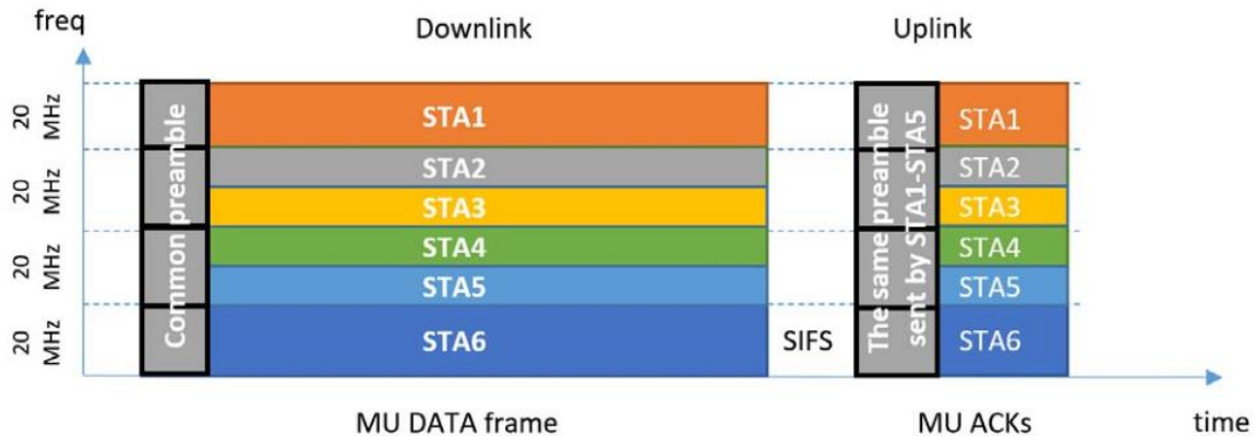
Slika 8. Prikaz OFDMA prijensa u 802.11ax, [7]
