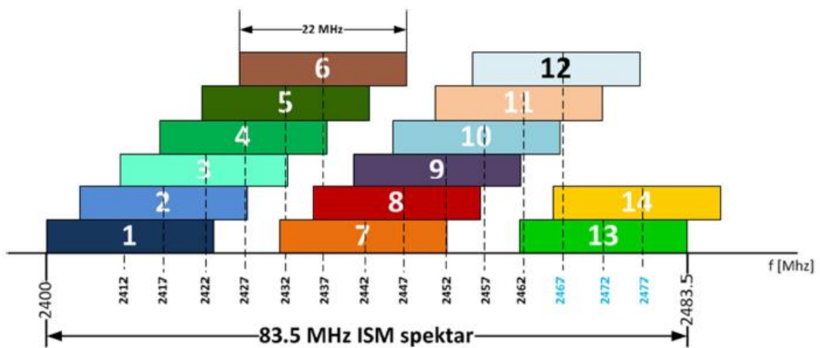
Slika 6. Raspored kanala u 2,4 GHz pojasu, [15].
