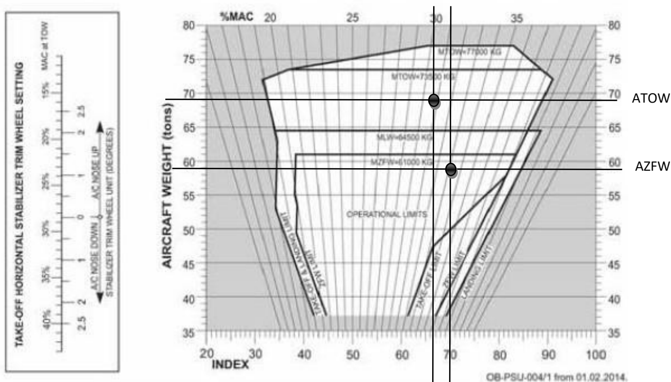
Slika 18. Balansni dijagram
