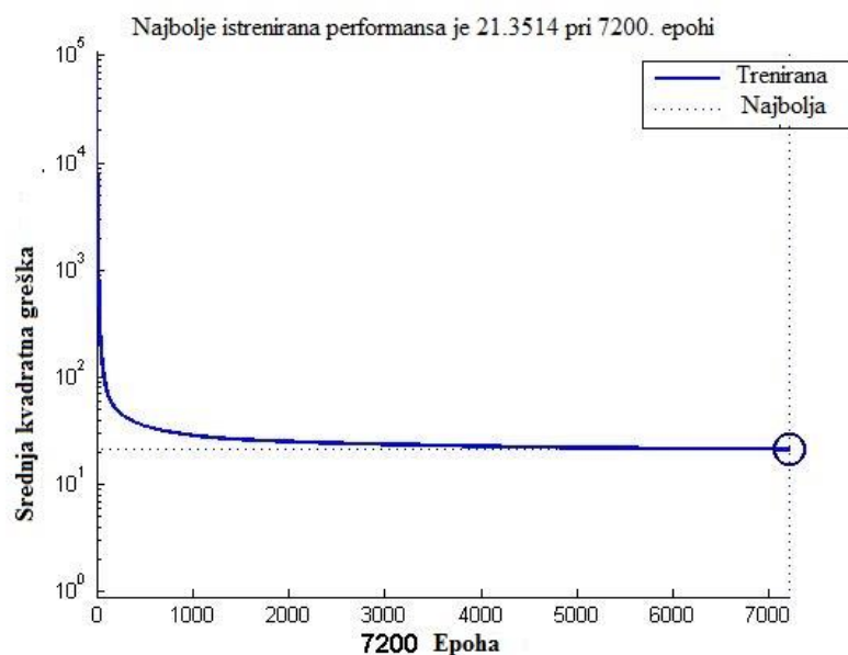
Slika 19: Prikaz odnosa performansi neuronske mreže i stupnja dobrote
