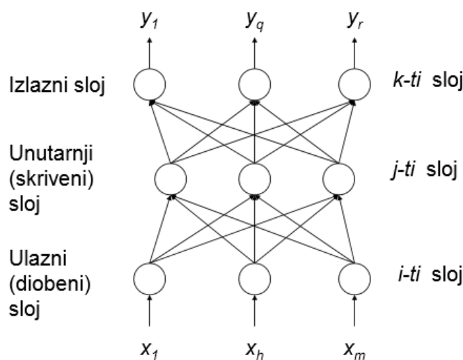
Slika 8: Arhitektura višeslojne mreže bez povratnih veza, [10]
