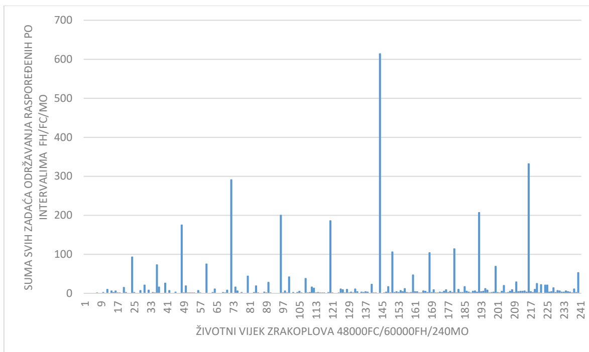
Graf 5. Raspored svih zadataka održavanja zrakoplova tijekom životnog vijeka koje se ponavljaju u intervalu većem od 12 mjeseci
