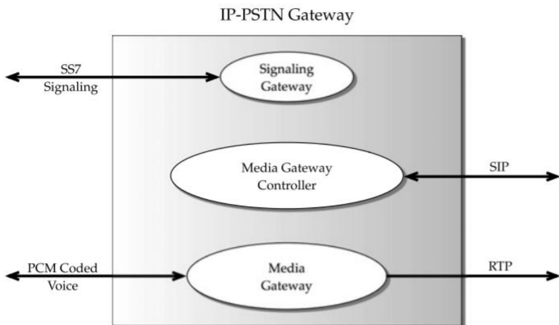
Slika 8. Gateway između PSTN i IP mreže, [1]
