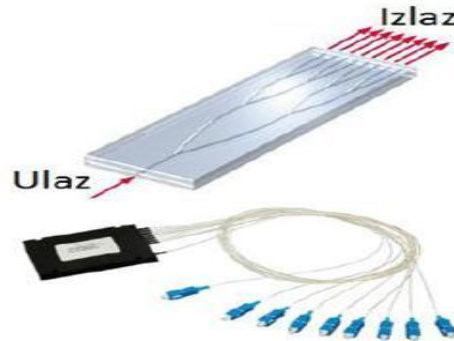
Slika 6 Primjer djelitelja [12]
