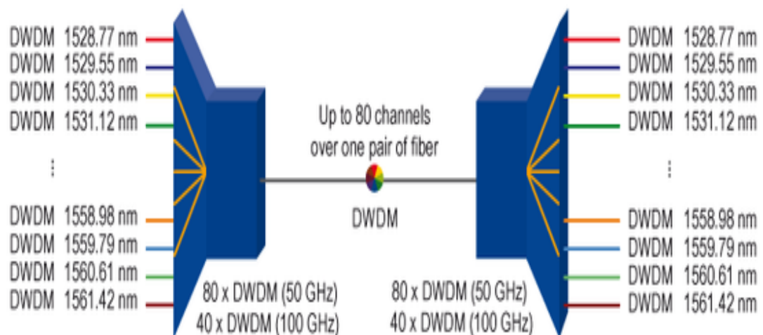
Slika 11 DWDM sustav [17]
