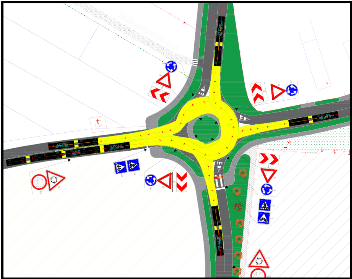
Slika 38. Provjerene trajektorije za rekonstruirano raskrižje u programskom alatu „AutoTURN“
