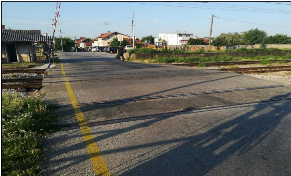
Slika 27. Prikaz stanja asfaltne podloge i drvenih pragova na željezničko-cestovnom prijelazu „Sokolska“
