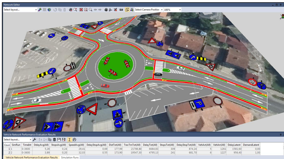
Slika 37. Prikaz simulacijskog modela prijedloga rješenja u programskom alatu PTV Vissim za raskrižje Sisačka ulica – Trg kralja Tomislava – Trg kralja Petra Krešimira IV.
