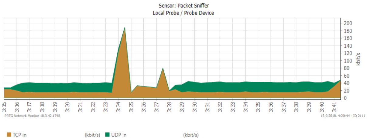
Slika 19: Brzina prijenosa dolaznog prometa u Prvom scenariju podijeljena na UDP i TCP promet
