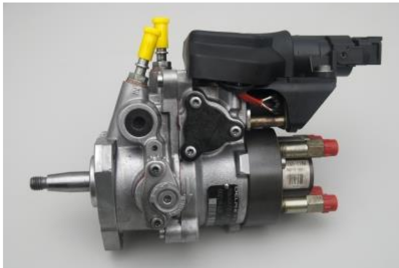
Slika 18. Potpuno elektronički upravljana radijalna visokotlačna pumpa [25]
