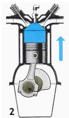
Slika 3. Drugi takt – kompresija [3]
