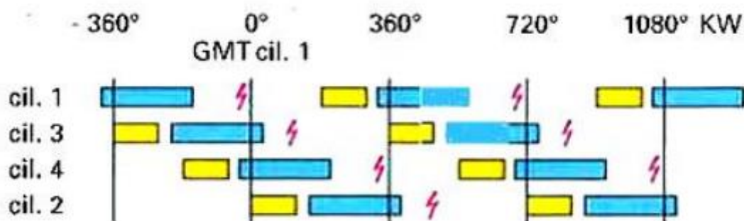
Slika 17. Slijedno ubrizgavanje
