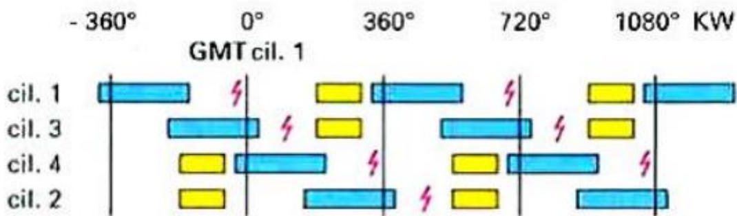
Slika 16. Grupno ubrizgavanje
