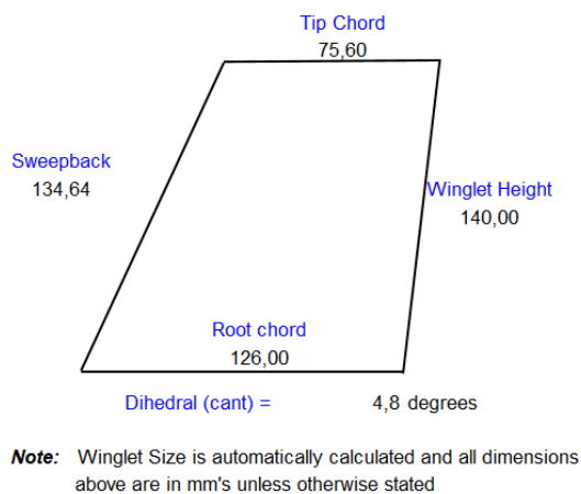
Slika 7 Prikaz dimenzija i izgled aerodinamičkih završetaka iz aplikacije Curtisa Sutera
