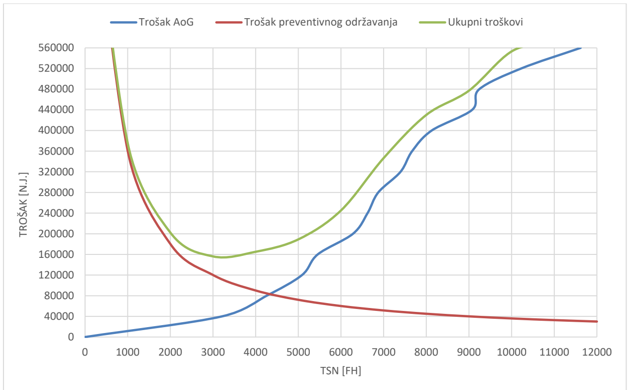
Graf 5: Odnos troškova AoG, troškova preventivnog održavanja te ukupnih troškova održavanja
