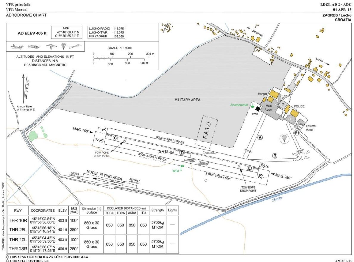
Slika 14: Tlocrt aerodroma Lučko [15]
