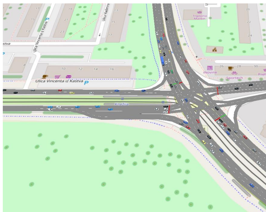
Slika 30 Isječak iz simulacije mreže nakon implementiranja rješenja na raskrižju Selska cesta - Horvaćanska cesta
