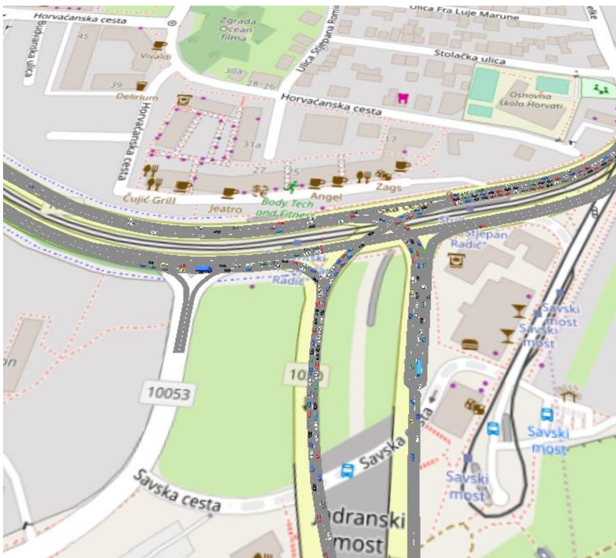
Slika 26 Simulacija raskrižja Selska cesta – Jadranski most nakon implementiranog rješenja
