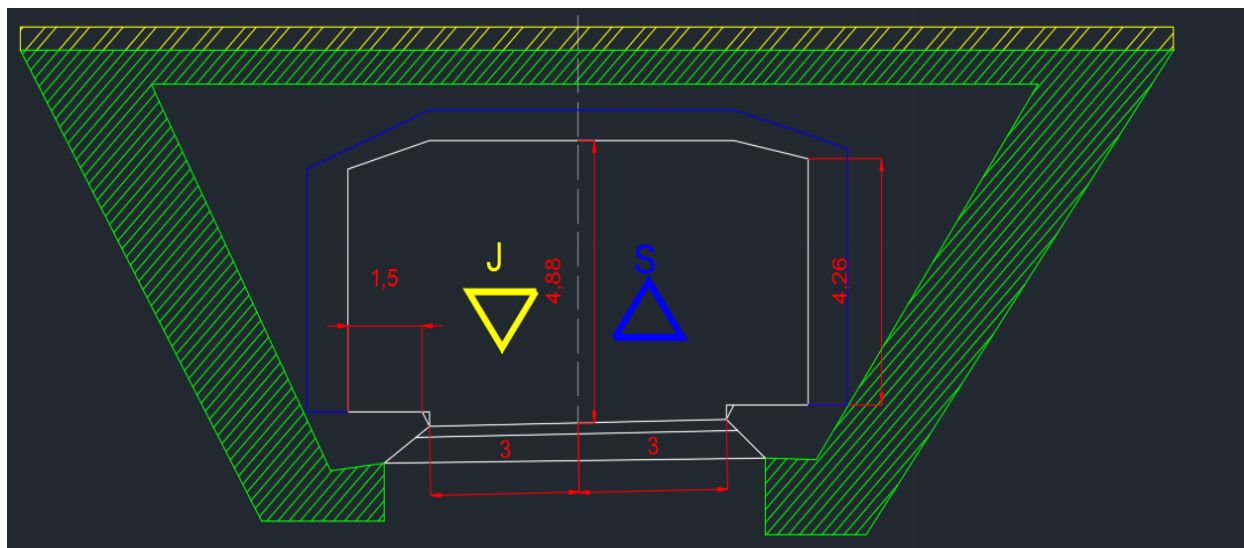
Slika 13. Poprečni presjek podvožnjaka
