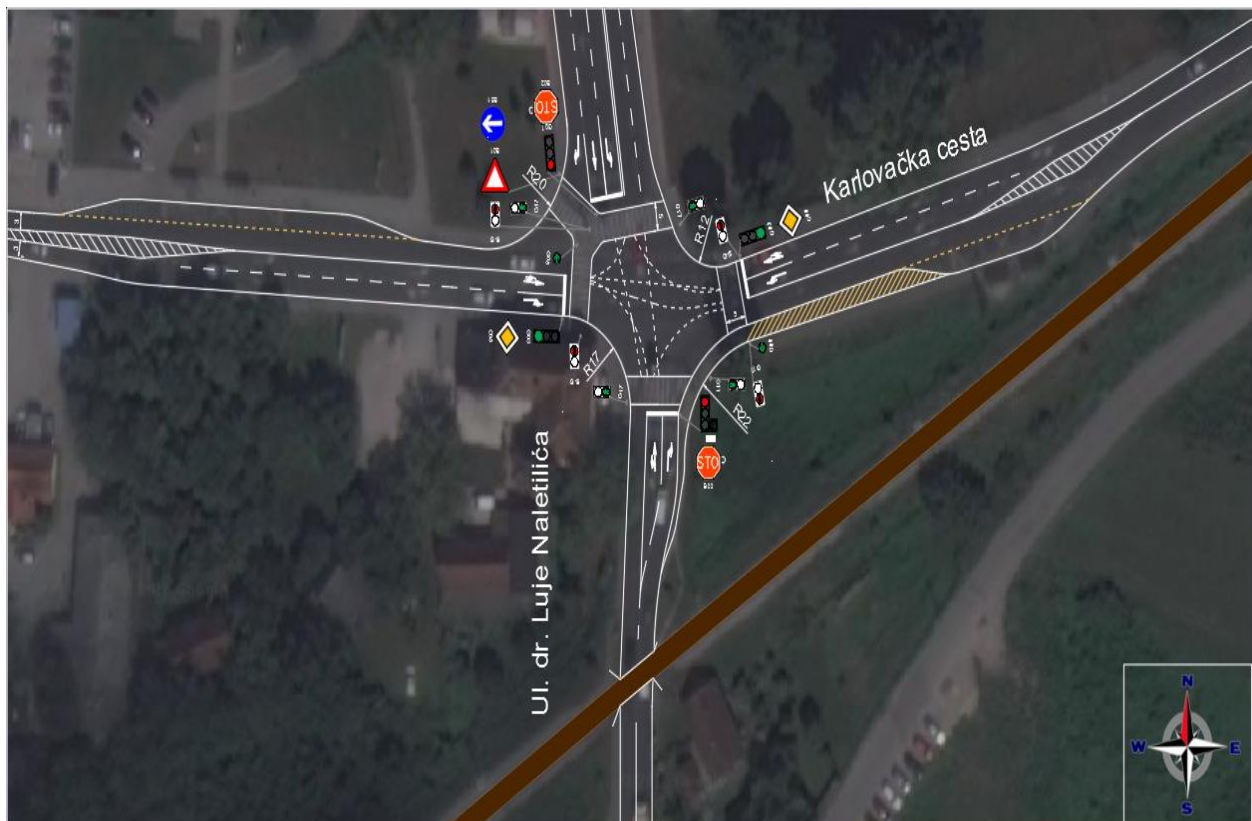
Slika 12. Shematski prikaz Varijante 2
