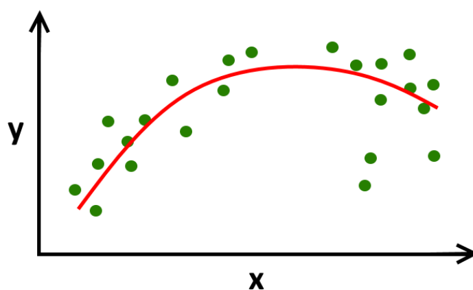
Slika 5.4: Regresija
