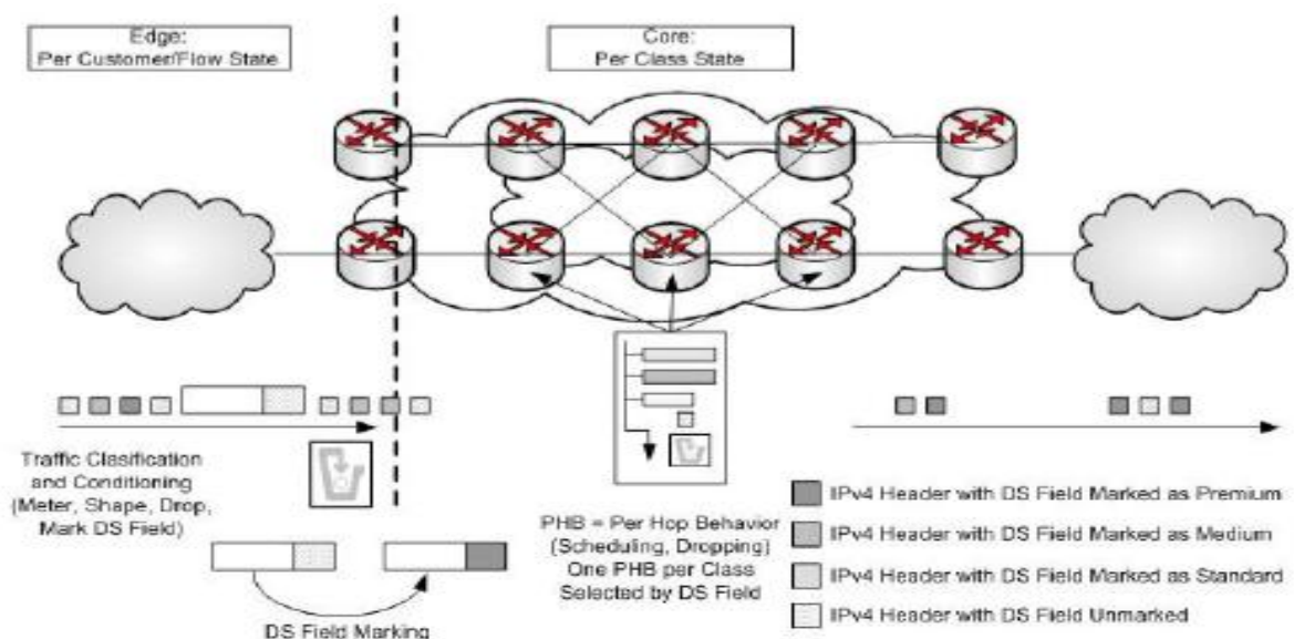
Slika 3. DiffServ arhitektura [4]
