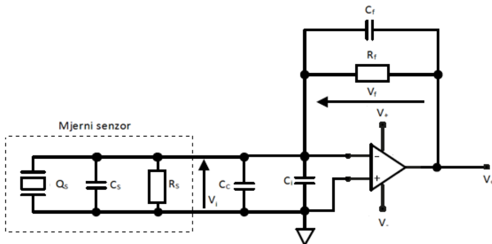
Slika 3.5. Shema konfiguracije nabojnog pojačala [4]
